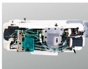
微油润滑系统 Semi oil lubrication system
